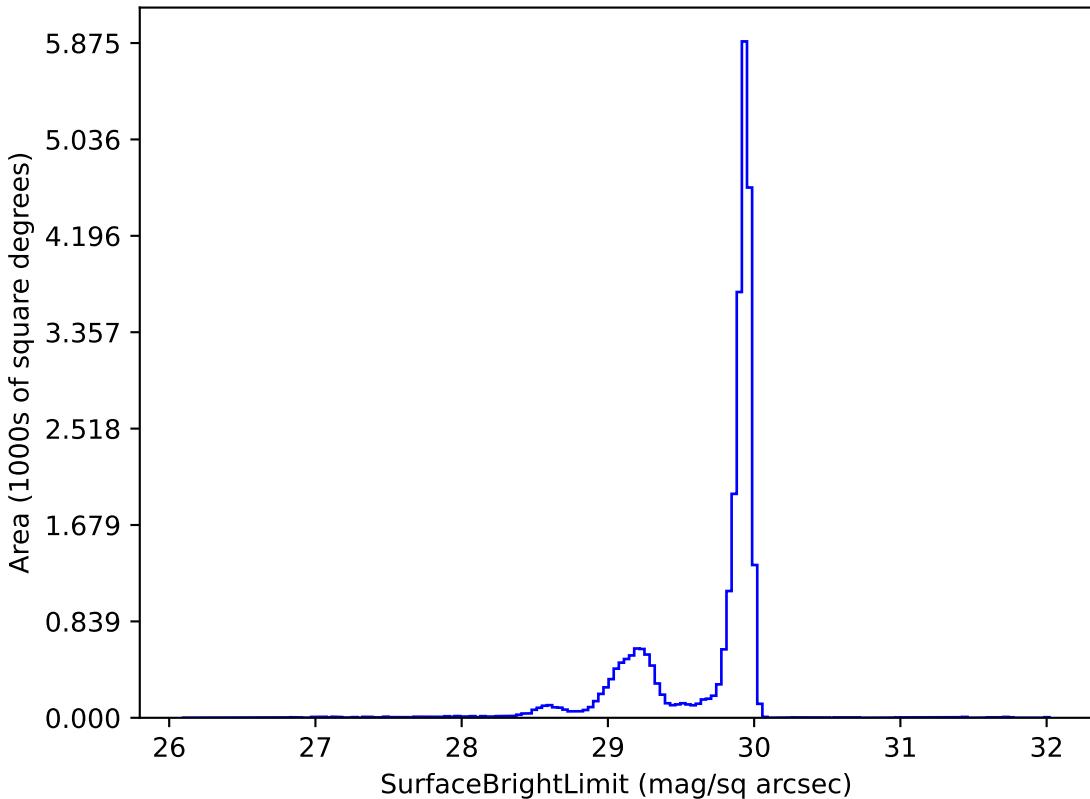
roman_v3.3_10yrs i: SurfaceBrightLimit
