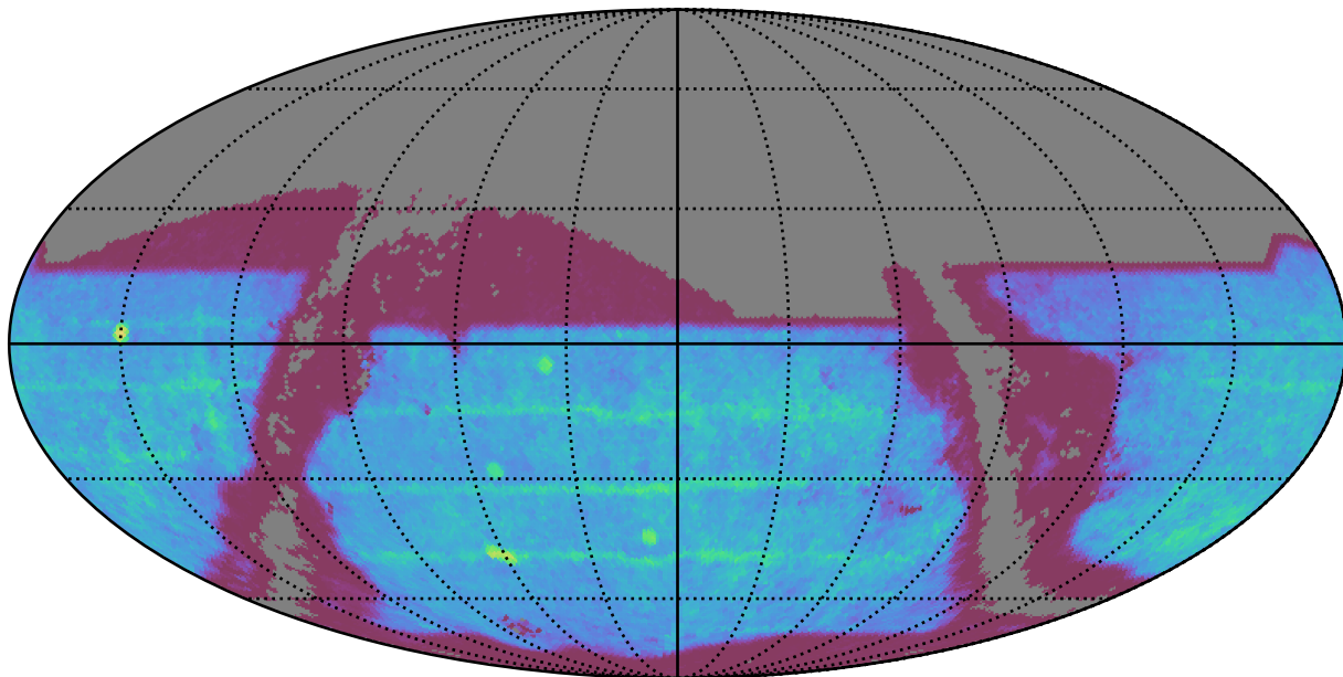
roman_v3.3_10yrs : SNSLMetric
