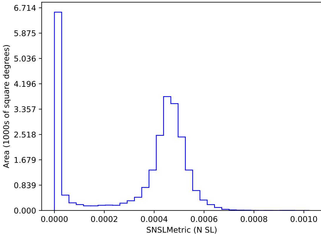
roman_v3.3_10yrs : SNSLMetric
