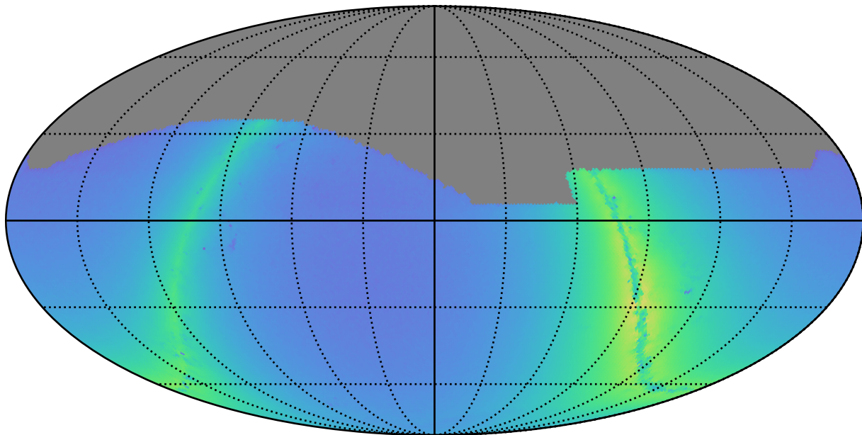
roman_v3.3_10yrs i: Nstars_no_crowding
