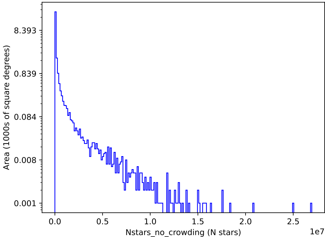
roman_v3.3_10yrs i: Nstars_no_crowding
