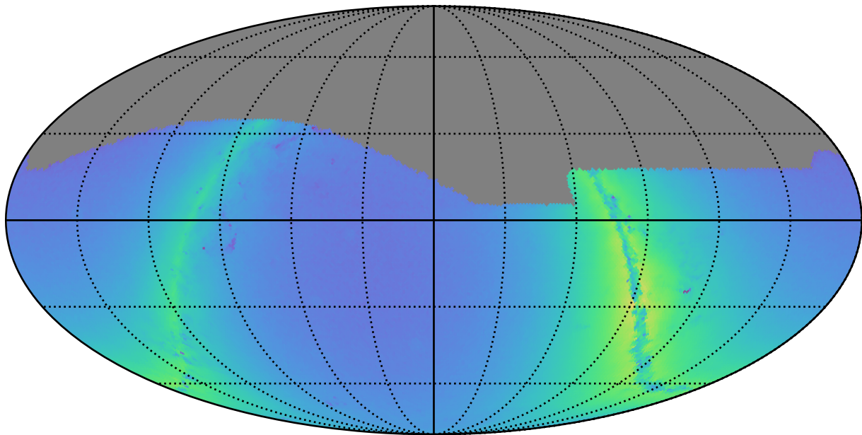
roman_v3.3_10yrs g:Nstars_no_crowding
