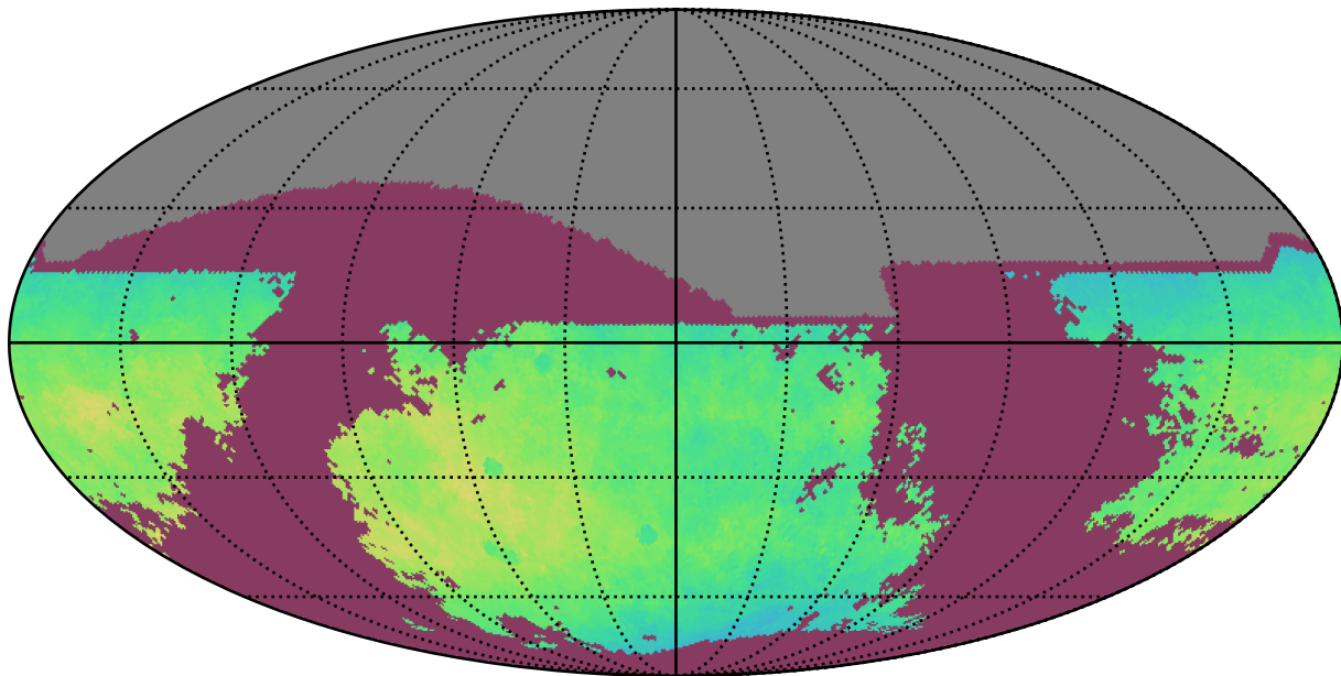
roman_v3.3_10yrs i: NgalScale
