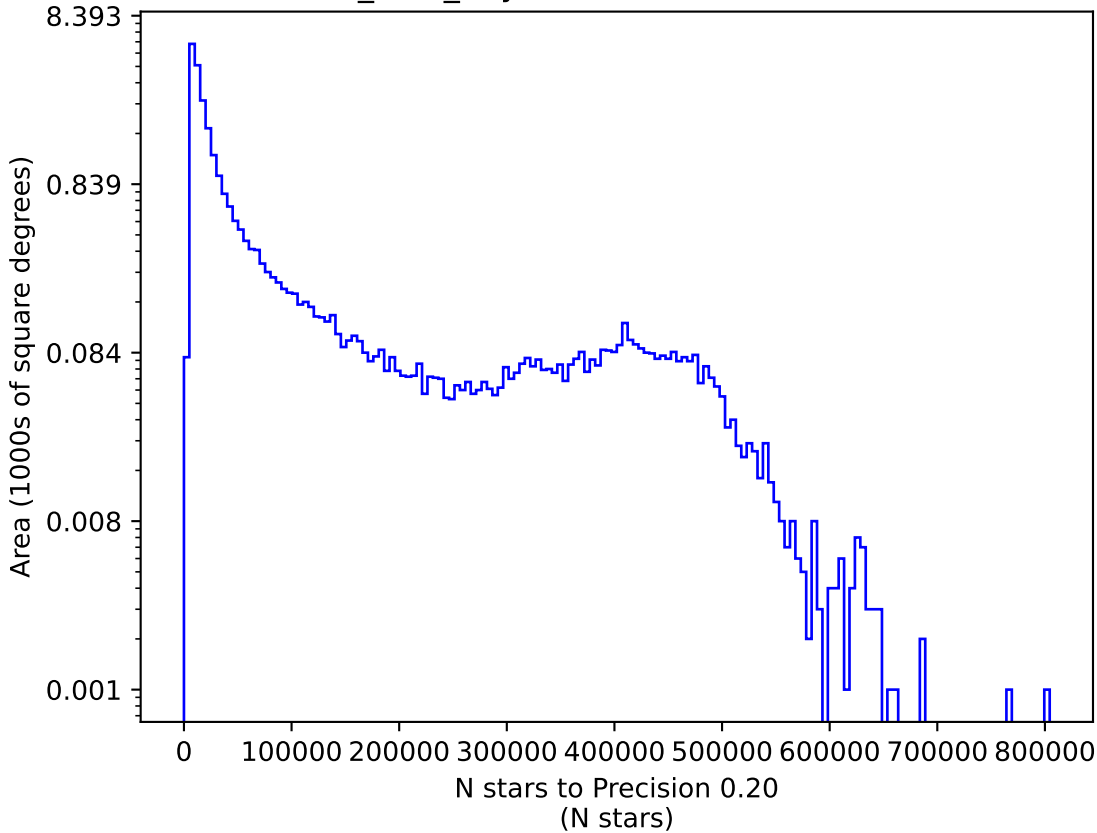
roman_v3.3_10yrs i: N stars to Precision 0.20
