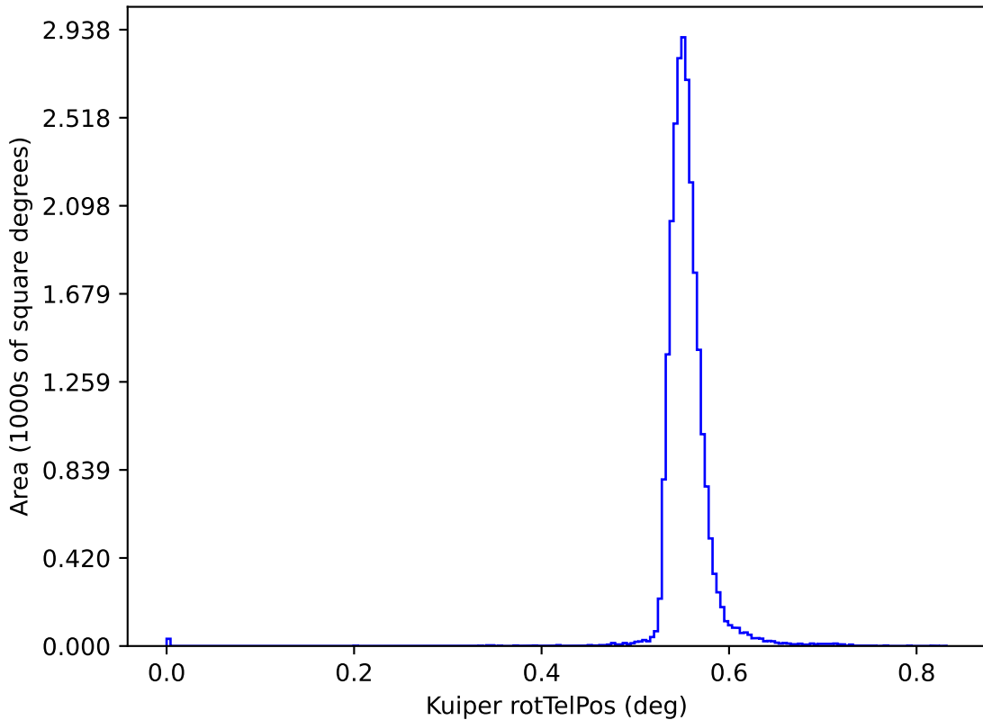
roman_v3.3_10yrs y: Kuiper rotTelPos
