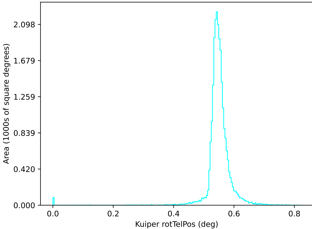
roman_v3.3_10yrs u: Kuiper rotTelPos
