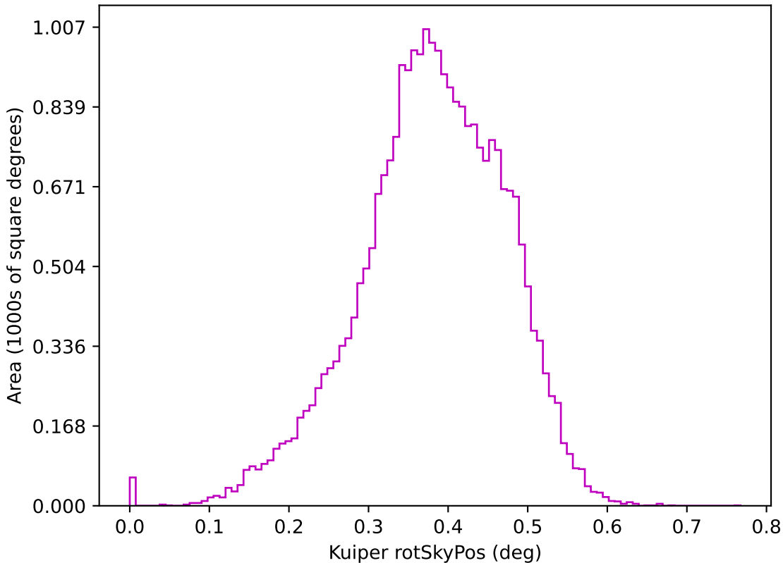
roman_v3.3_10yrs z: Kuiper rotSkyPos
