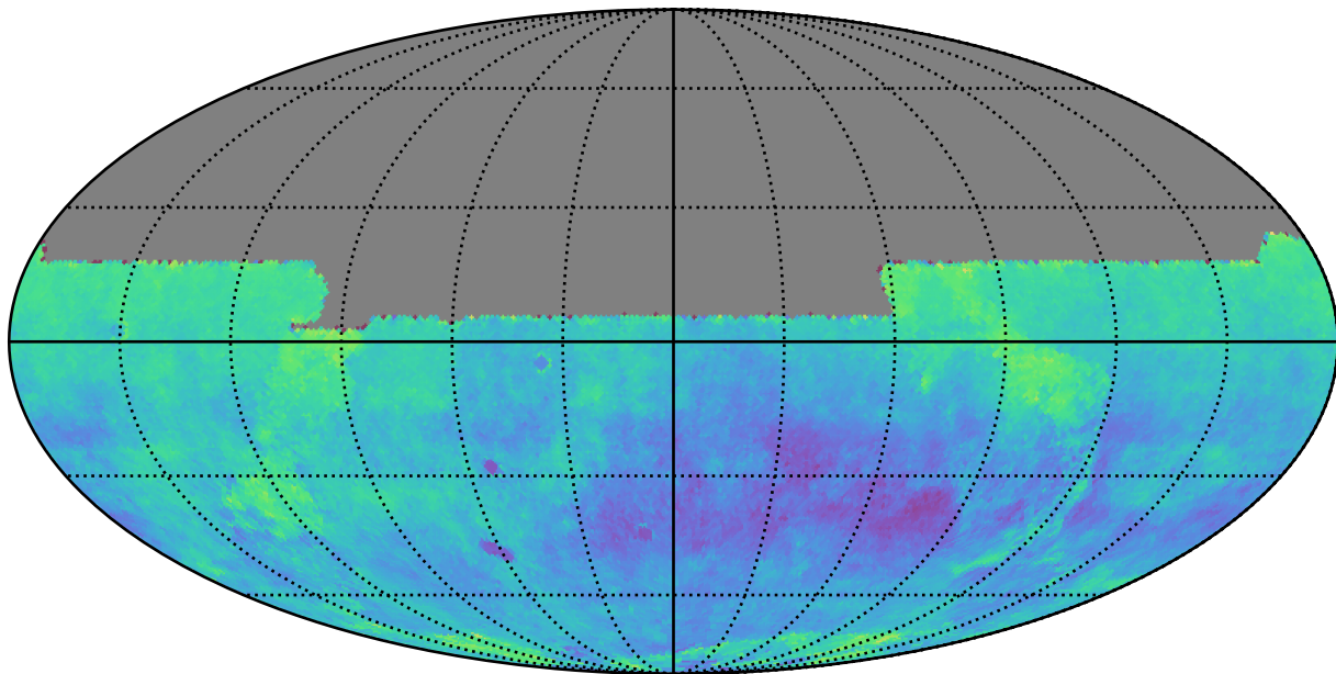
roman_v3.3_10yrs y: Kuiper rotSkyPos
