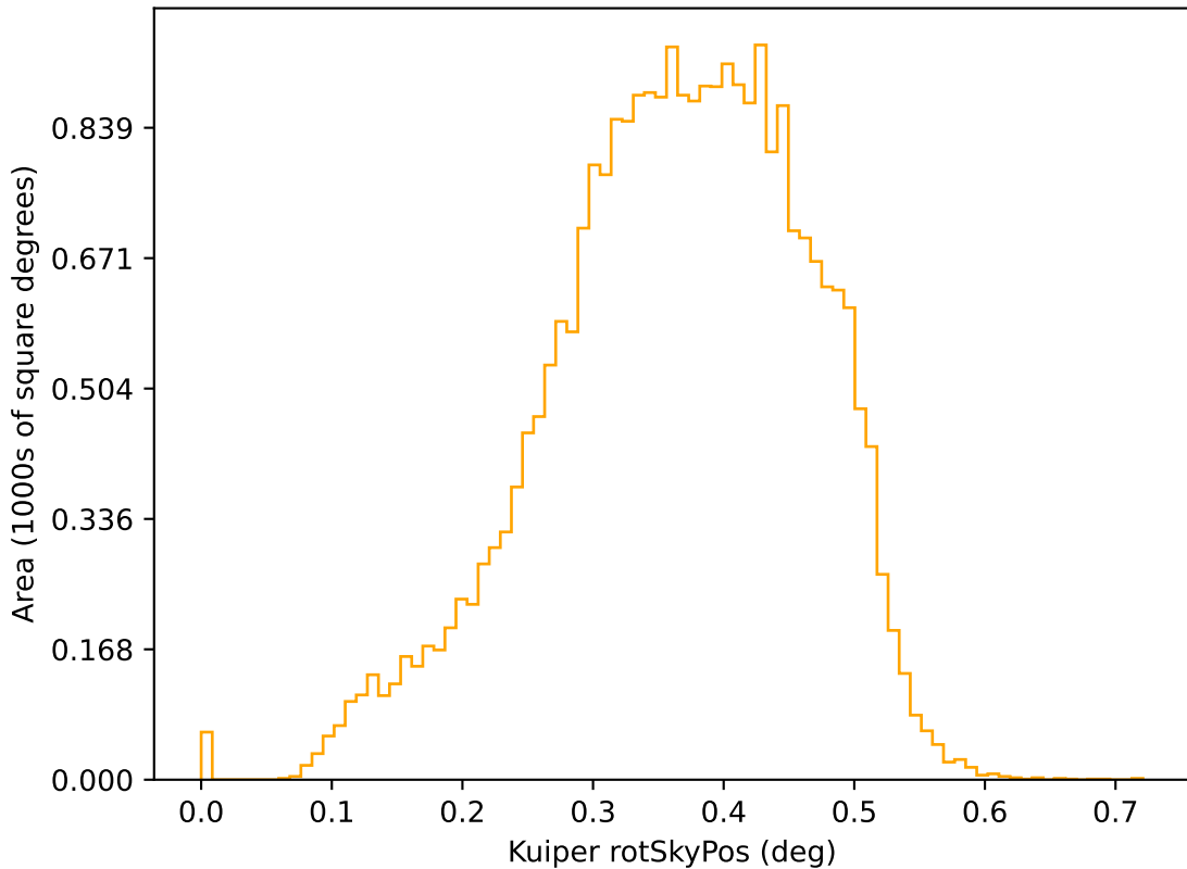
roman_v3.3_10yrs r: Kuiper rotSkyPos
