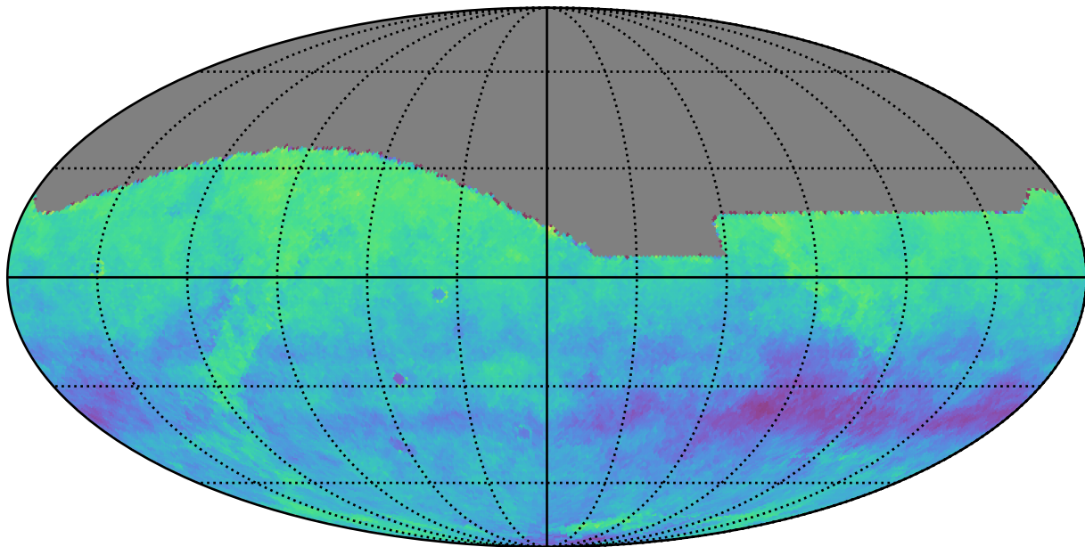
roman_v3.3_10yrs i: Kuiper rotSkyPos
