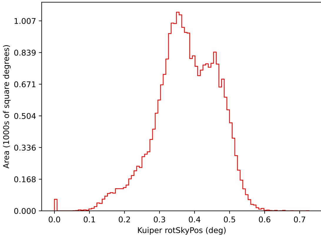
roman_v3.3_10yrs i: Kuiper rotSkyPos
