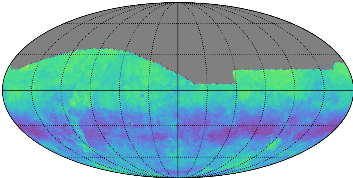
roman_v3.3_10yrs g: Kuiper rotSkyPos
