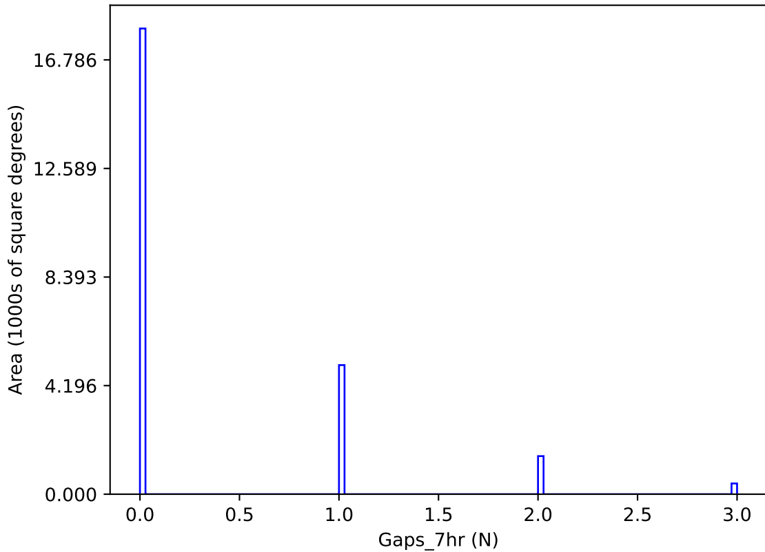
roman_v3.3_10yrs y band: Gaps_7hr
