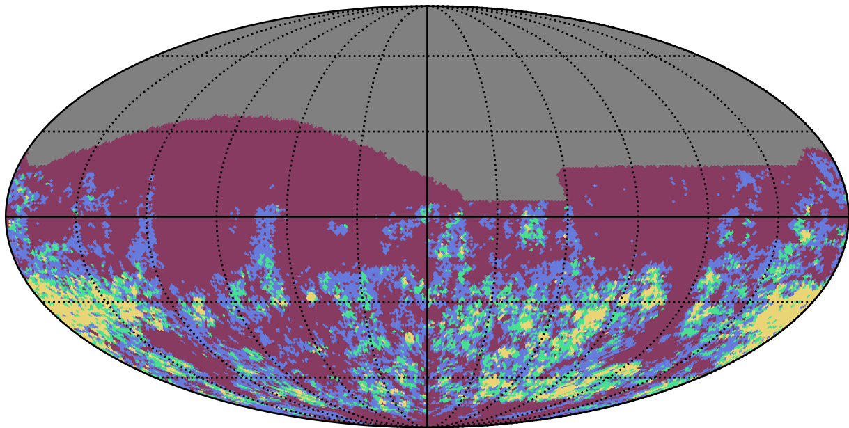
roman_v3.3_10yrs i band: Gaps_7hr
