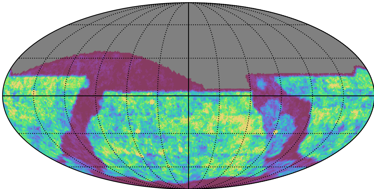
roman_v3.3_10yrs z band: Gaps_24hr
