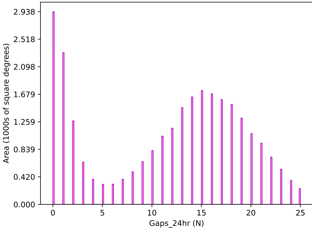
roman_v3.3_10yrs z band: Gaps_24hr
