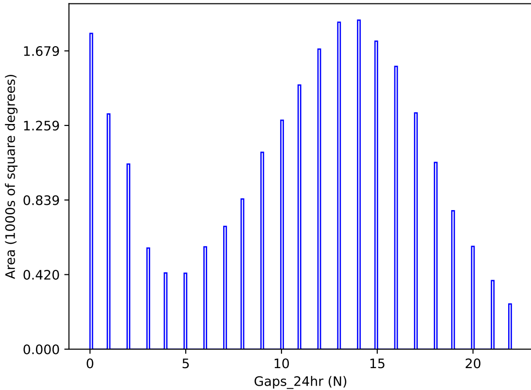
roman_v3.3_10yrs y band: Gaps_24hr
