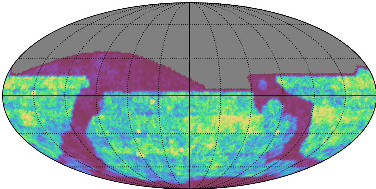
roman_v3.3_10yrs i band: Gaps_24hr
