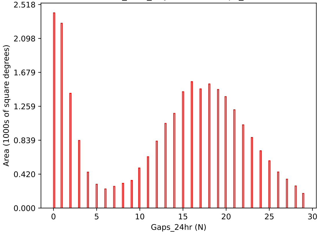
roman_v3.3_10yrs i band: Gaps_24hr
