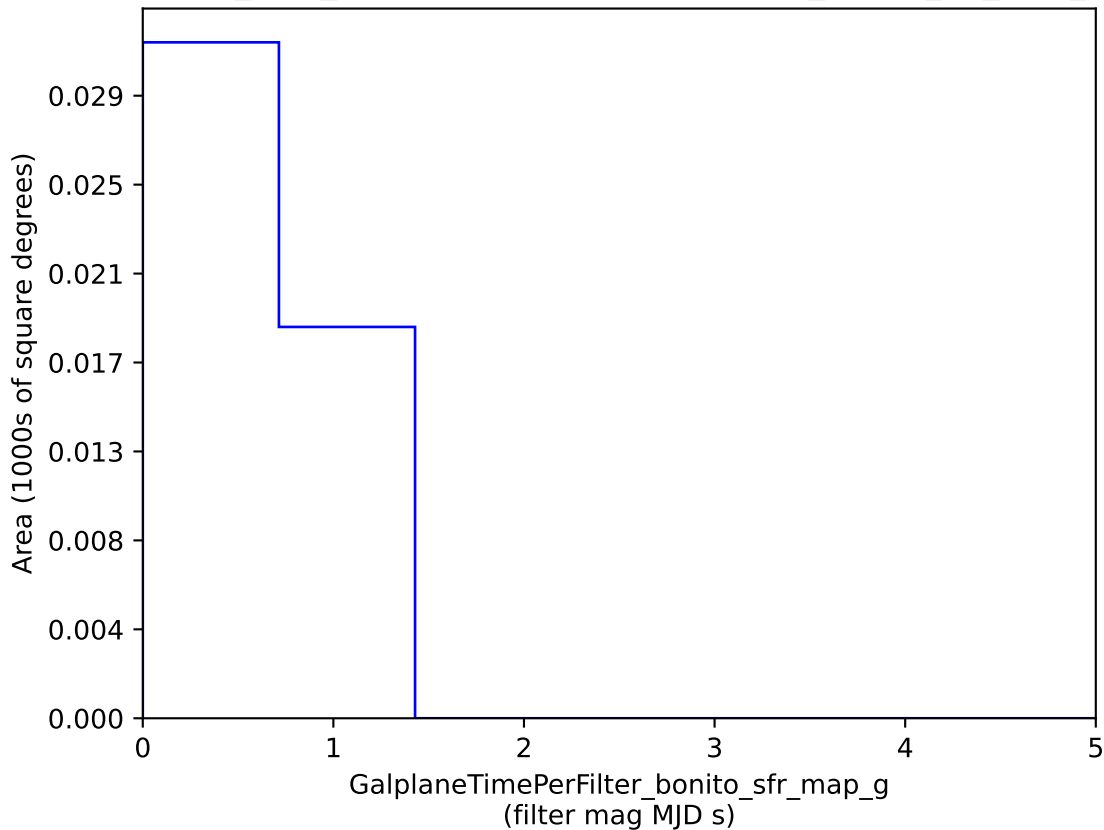
roman_v3.3_10yrs : GalplaneTimePerFilter_bonito_sfr_map_g
