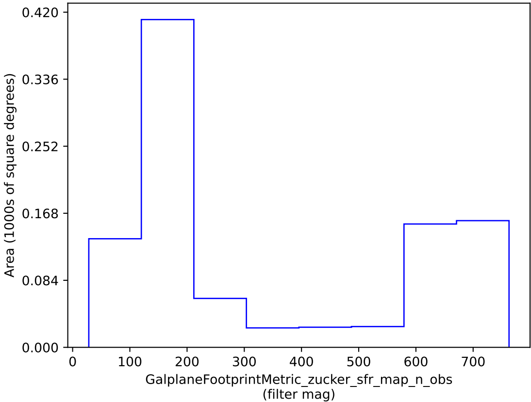
roman_v3.3_10yrs : GalplaneFootprintMetric_zucker_sfr_map_n_obs
