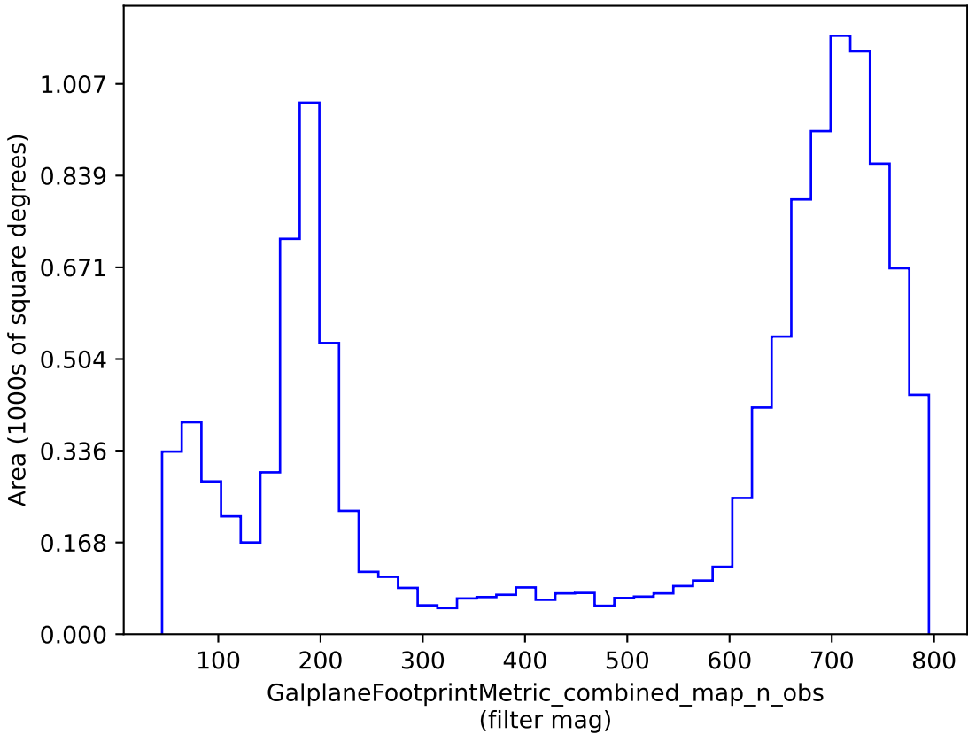
roman_v3.3_10yrs : GalplaneFootprintMetric_combined_map_n_obs
