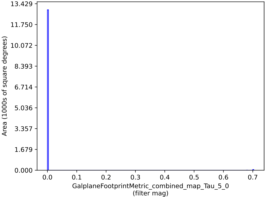
roman_v3.3_10yrs : GalplaneFootprintMetric_combined_map_Tau_5_0
