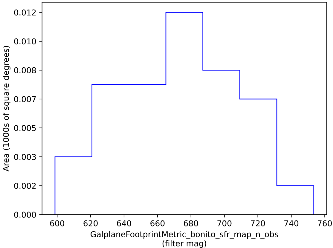
roman_v3.3_10yrs : GalplaneFootprintMetric_bonito_sfr_map_n_obs
