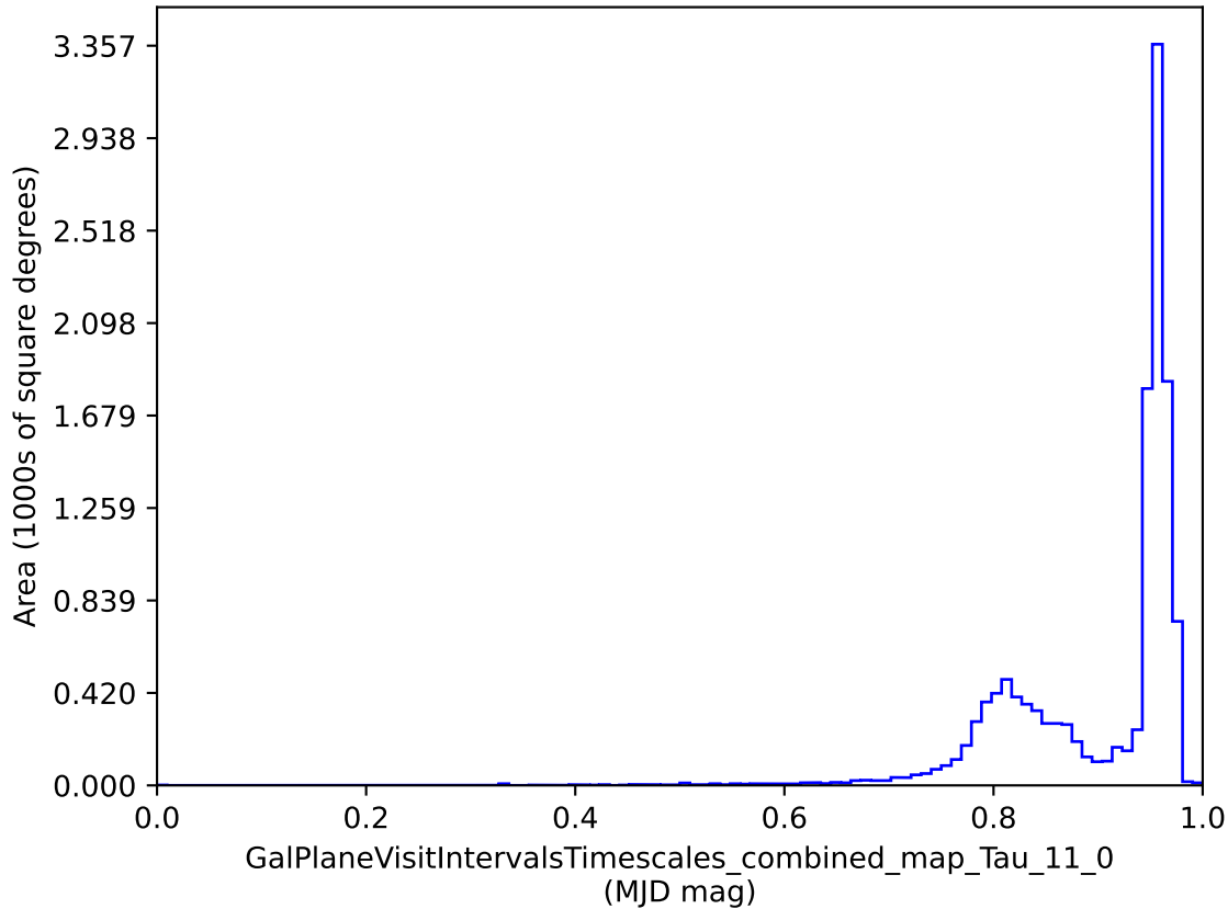
roman_v3.3_10yrs : GalPlaneVisitIntervalsTimescales_combined_map_Tau_11_0
