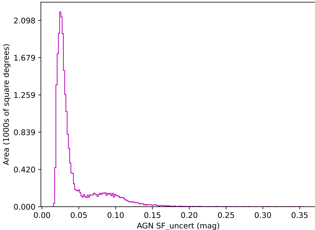
roman_v3.3_10yrs z band: AGN SF_uncert
