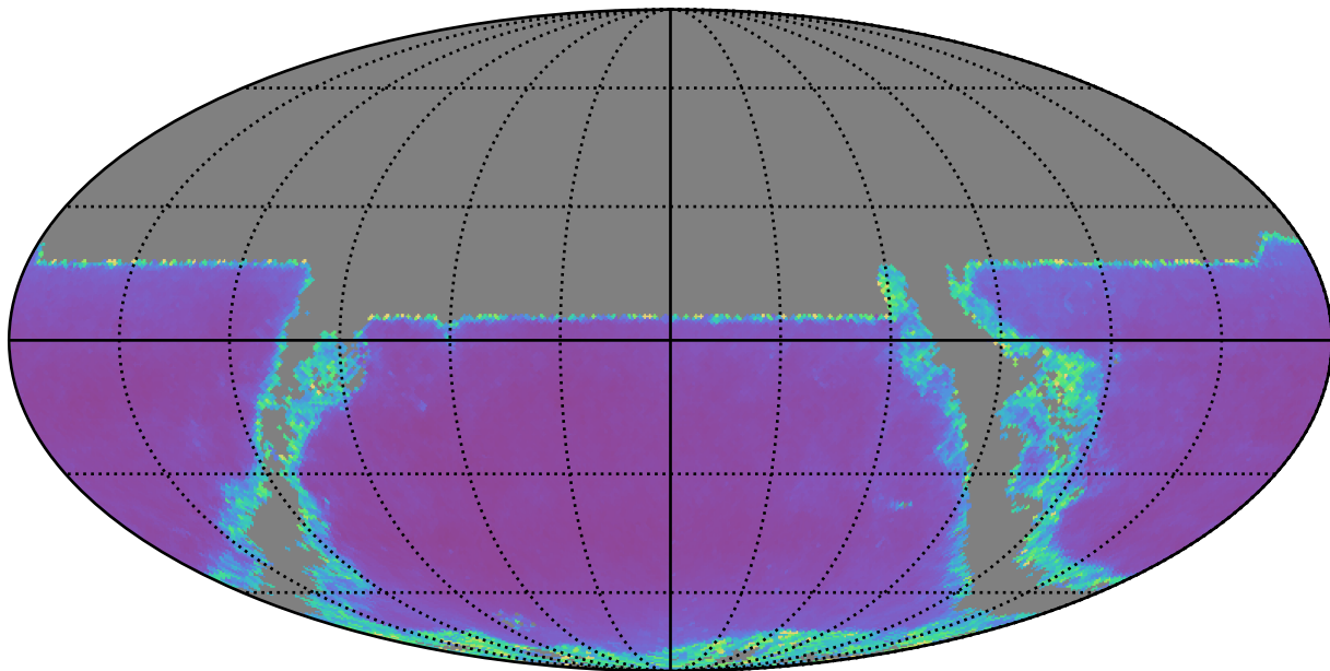
roman_v3.3_10yrs y band: AGN SF_uncert
