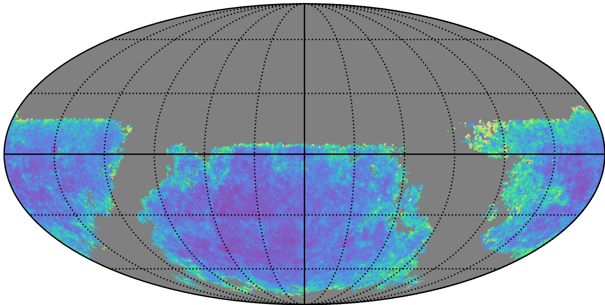
roman_v3.3_10yrs u band: AGN SF_uncert
