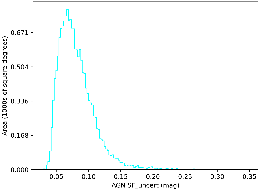
roman_v3.3_10yrs u band: AGN SF_uncert
