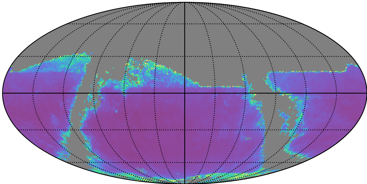
roman_v3.3_10yrs r band: AGN SF_uncert
