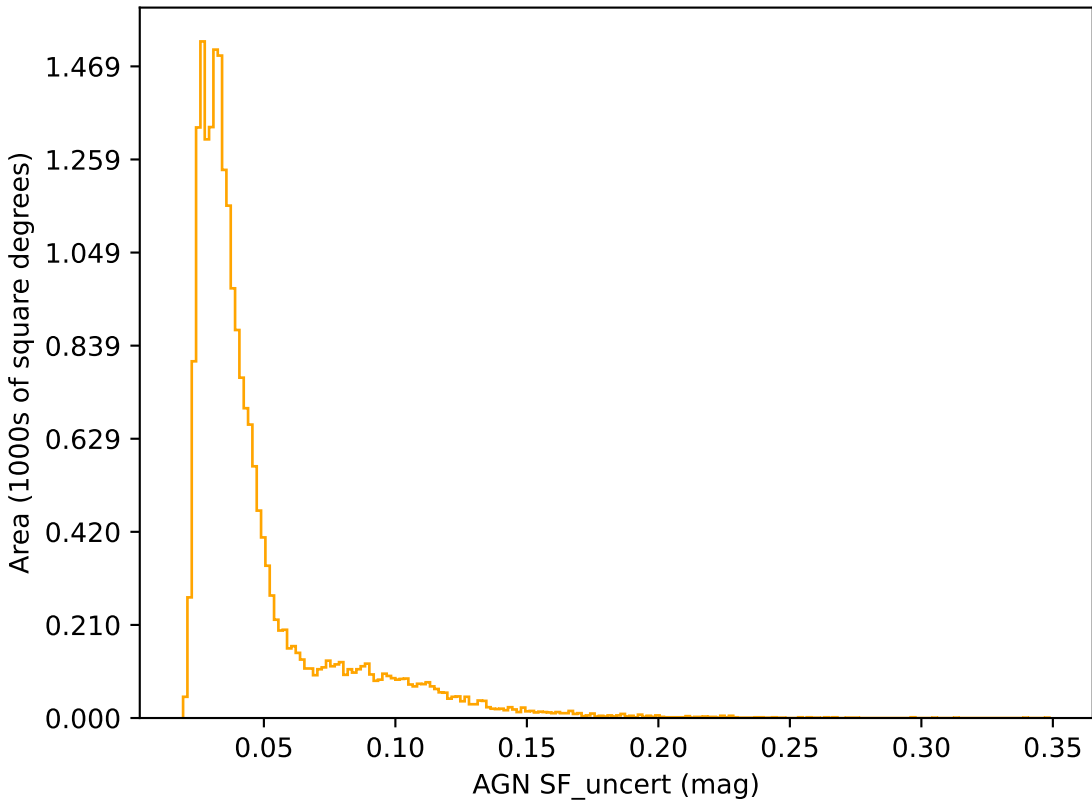
roman_v3.3_10yrs r band: AGN SF_uncert
