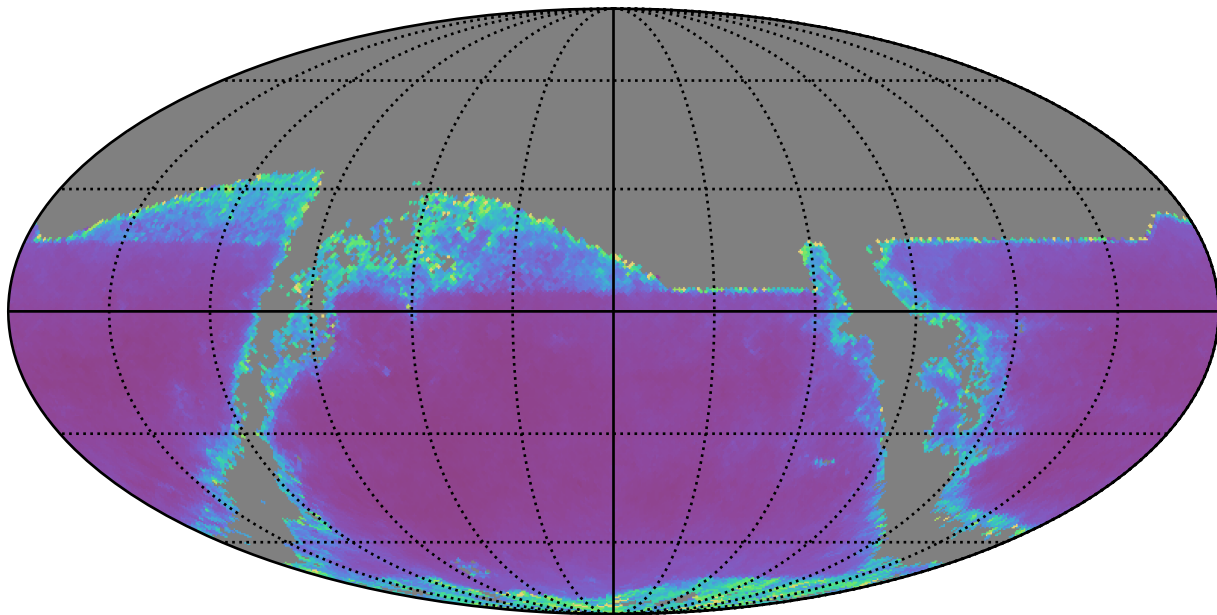
roman_v3.3_10yrs i band: AGN SF_uncert
