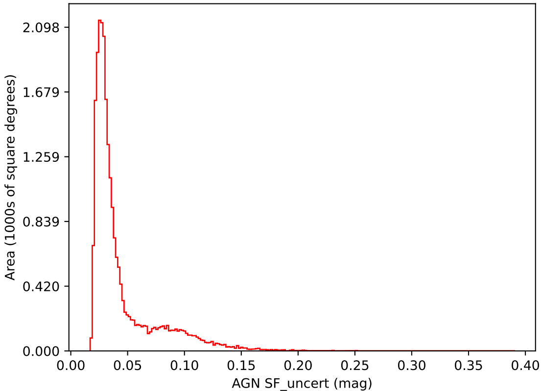
roman_v3.3_10yrs i band: AGN SF_uncert
