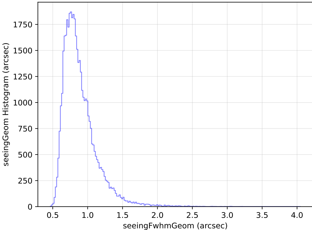
roman_v3.3_10yrs Yr 1 z band: seeingGeom Histogram
