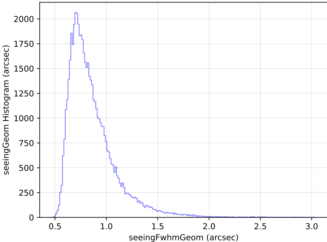
roman_v3.3_10yrs Yr 1 i band: seeingGeom Histogram
