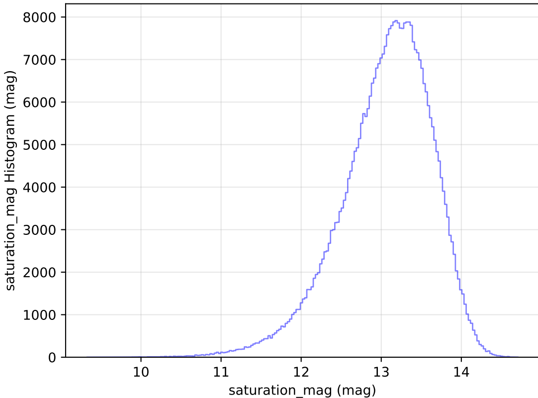
roman_v3.3_10yrs WFD y band: saturation_mag Histogram
