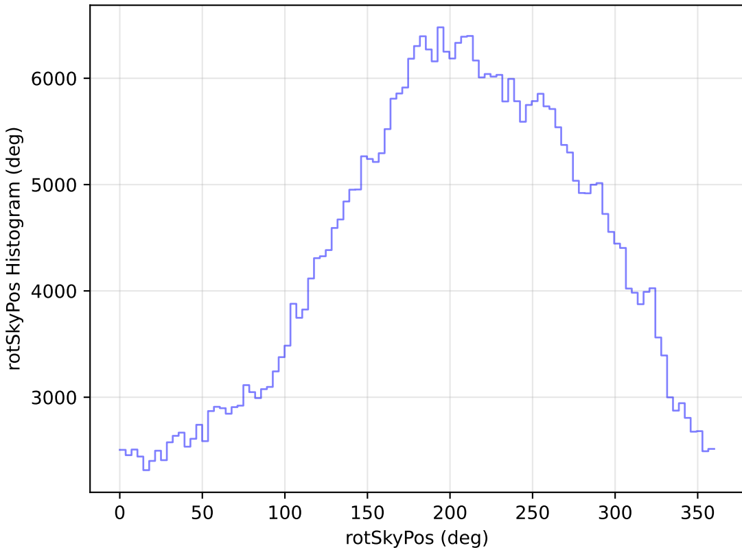
roman_v3.3_10yrs WFD z band: rotSkyPos Histogram
