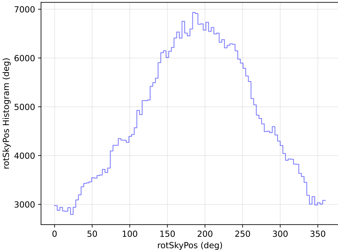
roman_v3.3_10yrs WFD r band: rotSkyPos Histogram
