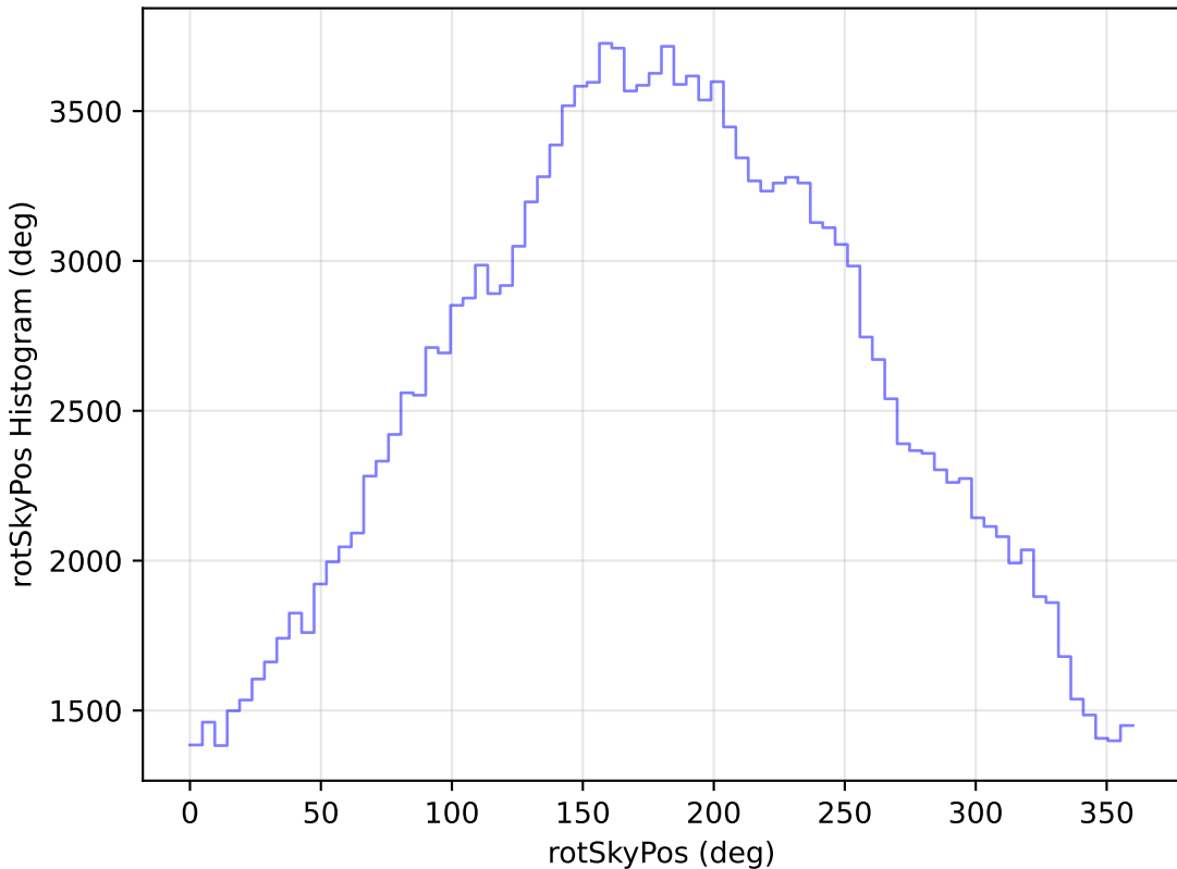
roman_v3.3_10yrs WFD g band: rotSkyPos Histogram
