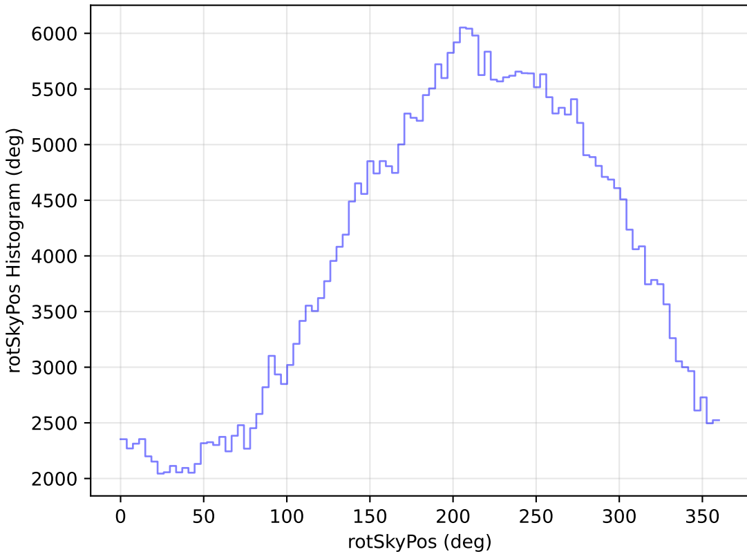
roman_v3.3_10yrs All sky y band: rotSkyPos Histogram
