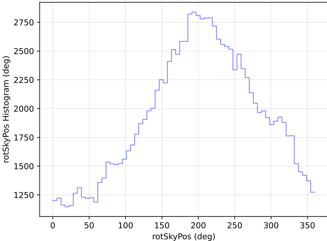
roman_v3.3_10yrs All sky u band: rotSkyPos Histogram
