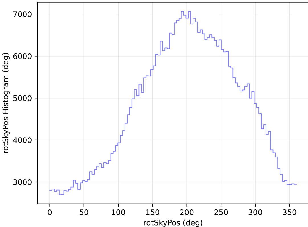
roman_v3.3_10yrs All sky i band: rotSkyPos Histogram
