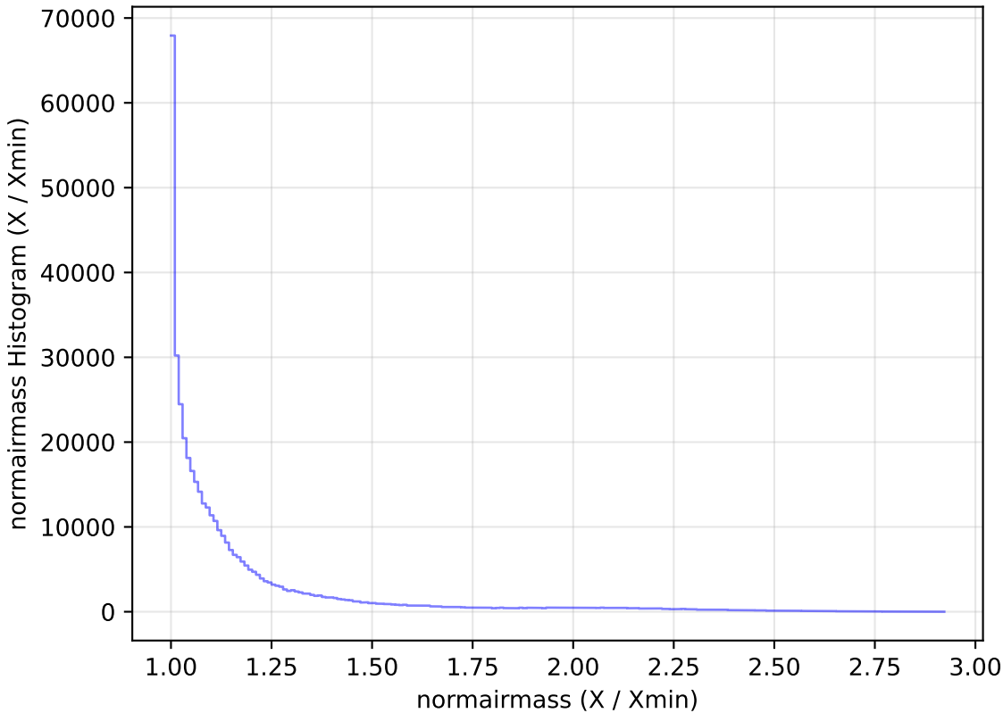
roman_v3.3_10yrs WFD z band: normairmass Histogram
