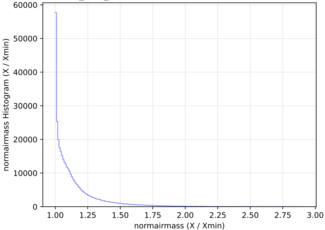
roman_v3.3_10yrs WFD y band: normairmass Histogram
