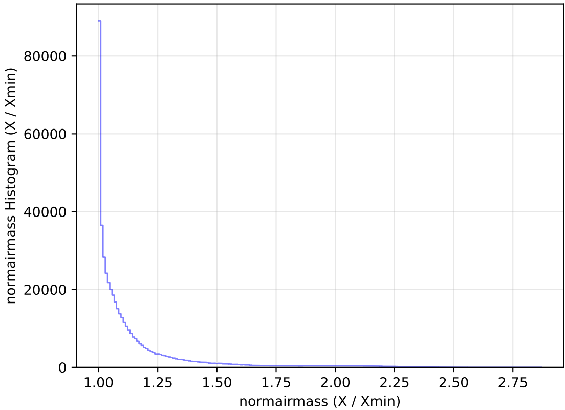
roman_v3.3_10yrs WFD r band: normairmass Histogram
