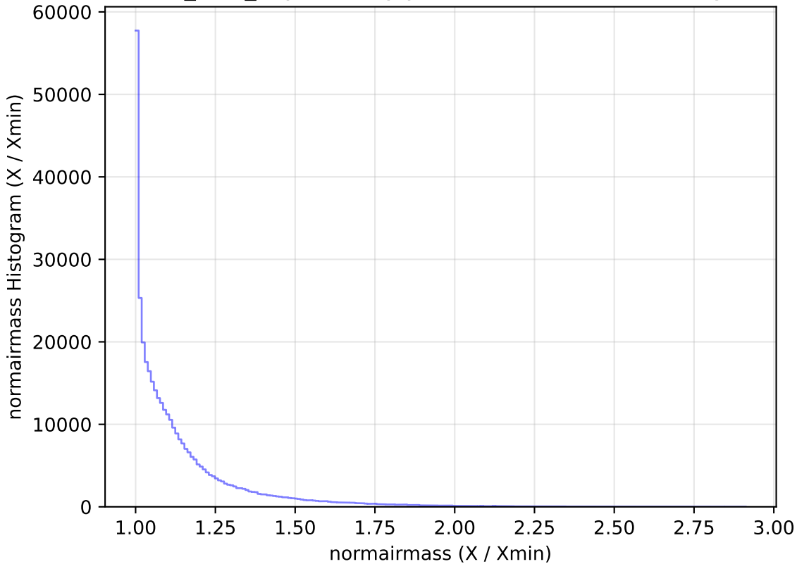
roman_v3.3_10yrs All sky y band: normairmass Histogram
